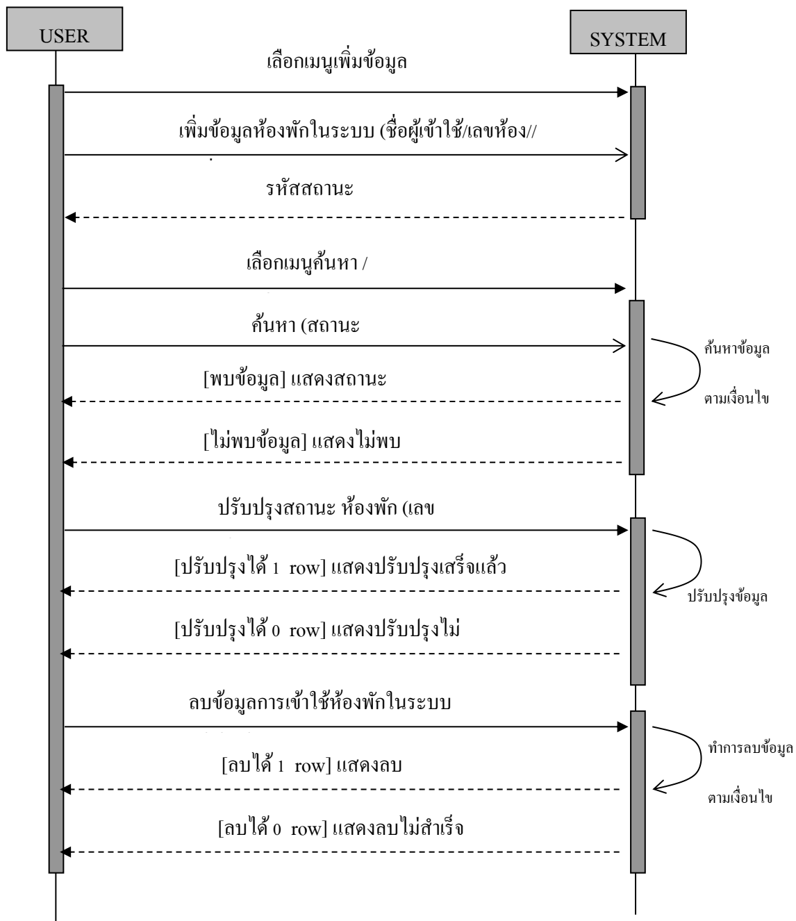
ตัวอย่าง SEQUENCE DIAGRAM ของ UC-02 ( ..... )
